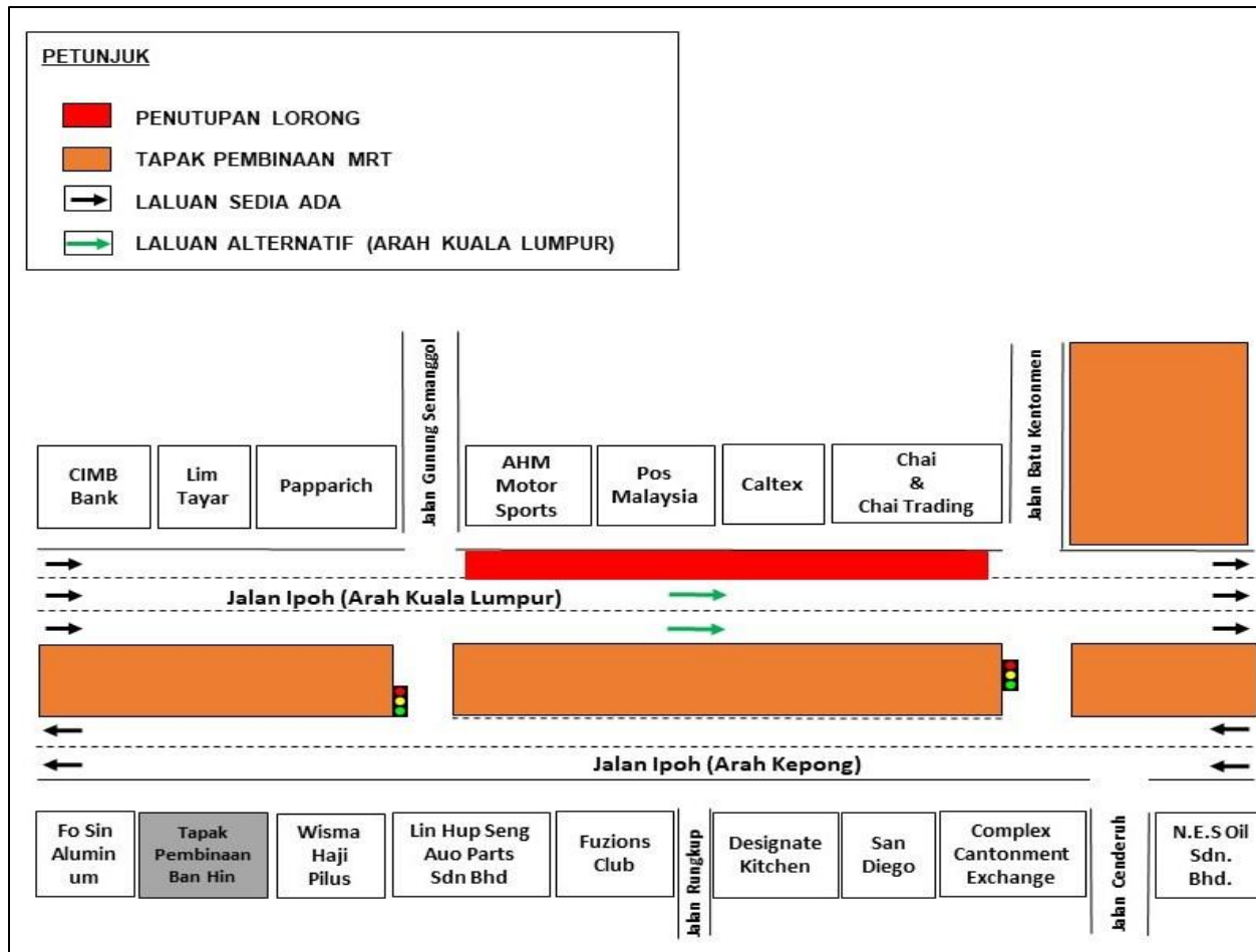
PETA 2B (PERINGKAT 2) : PENUTUPAN LORONG SECARA BERPERINGKAT DI JALAN IPOH (ARAH KUALA LUMPUR) SELEPAS PERSIMPANGAN LAMPU ISYARAT JALAN GUNUNG SEMANGGOL HINGGA KE PERSIMPANGAN LAMPU ISYARAT JALAN BATU KENTONMEN
