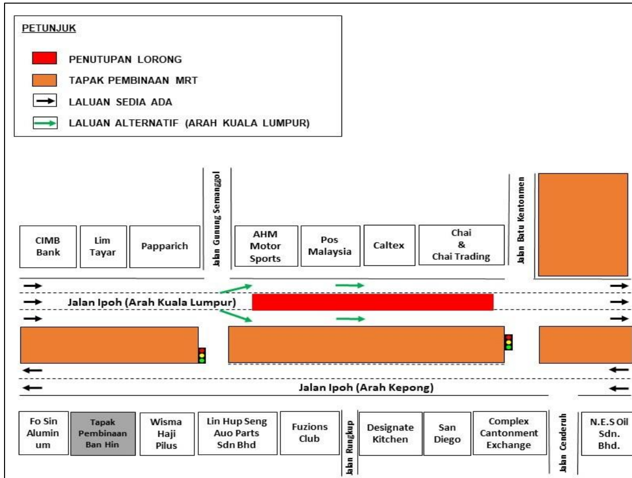
PETA 2A (PERINGKAT 1) : PENUTUPAN LORONG SECARA BERPERINGKAT DI JALAN IPOH (ARAH KUALA LUMPUR) SELEPAS PERSIMPANGAN LAMPU ISYARAT JALAN GUNUNG SEMANGGOL HINGGA KE PERSIMPANGAN LAMPU ISYARAT JALAN BATU KENTONMEN
