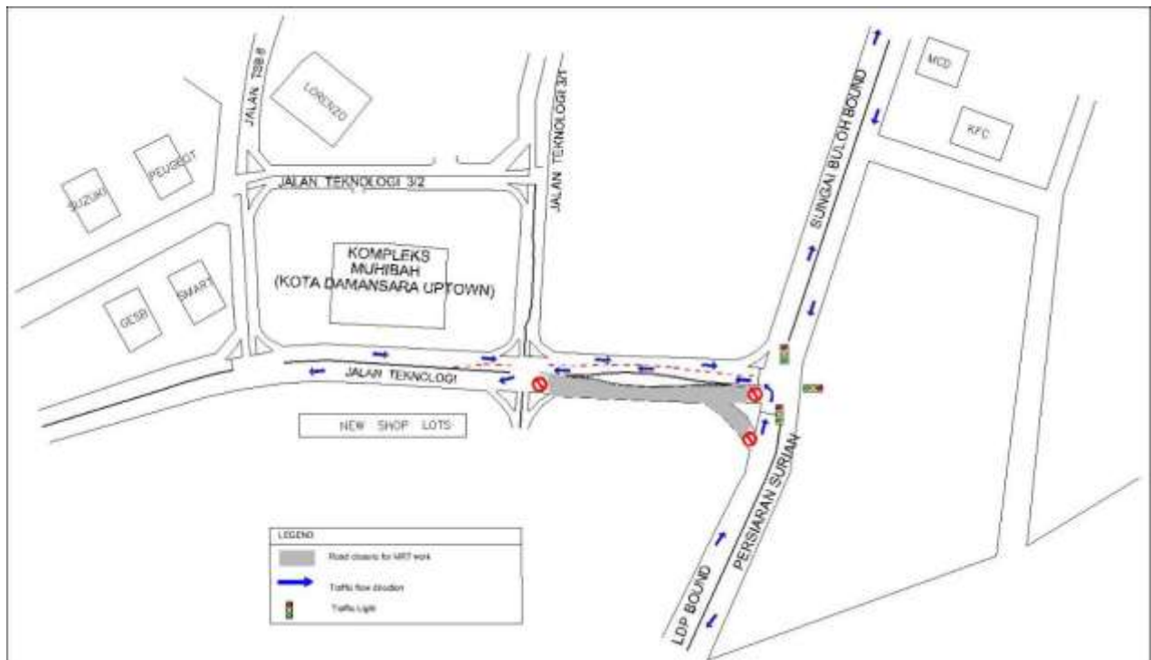
MAP 1 (B): TEMPORARY TRAFFIC CONTRA FLOW AT JALAN TEKNOLOGI / JALAN TEKNOLOGI 3/1 AND PERSIARAN SURIAN
